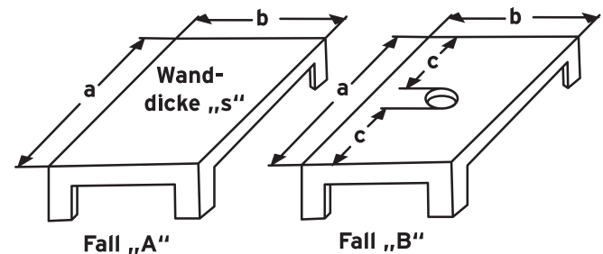
Bild 3: Beispiele für Wanddickentolerierung
