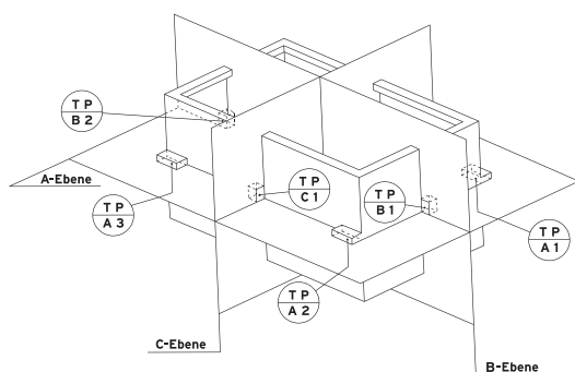
Bild 2: Bezugssystem (Schematisches Beispiel)
